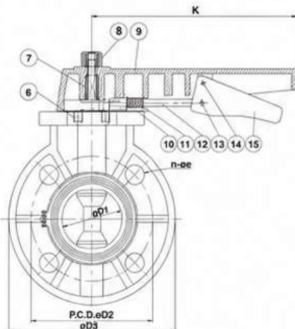
DN50~DN200
